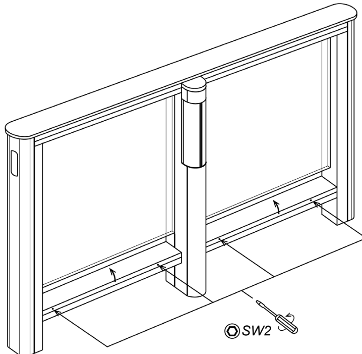
Рисунок 30. Снятие крышки нижнего короба
