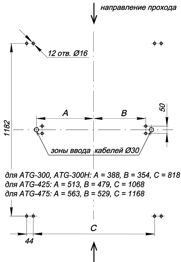
Рисунок 17. Схема разметки для монтажа турникета 1
