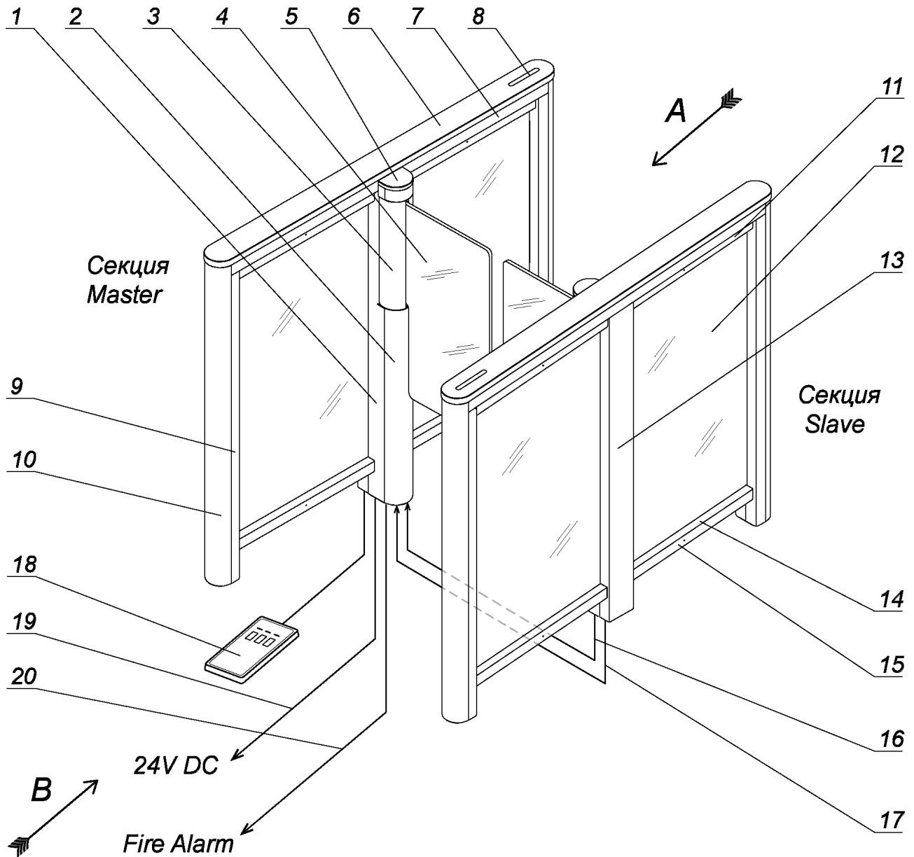
Рисунок 8. Внешний вид и устройство PERCo-ST-11:
