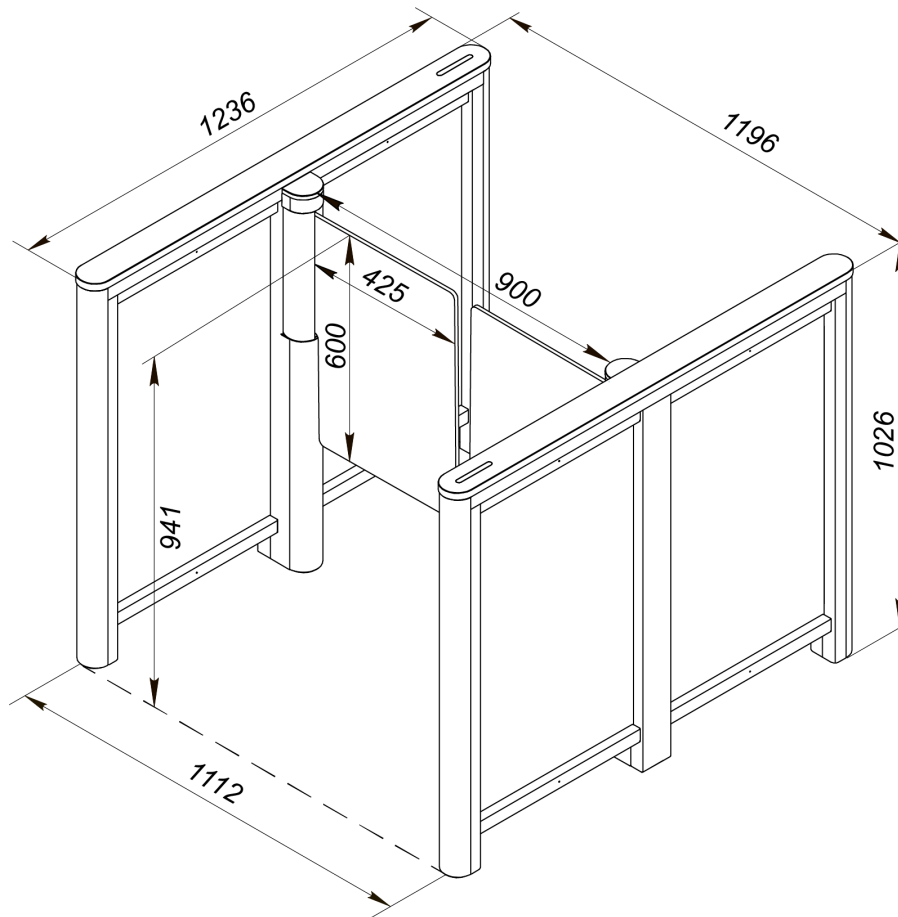
Рисунок 3. Габаритные размеры турникета со створками PERCo-ATG-425
