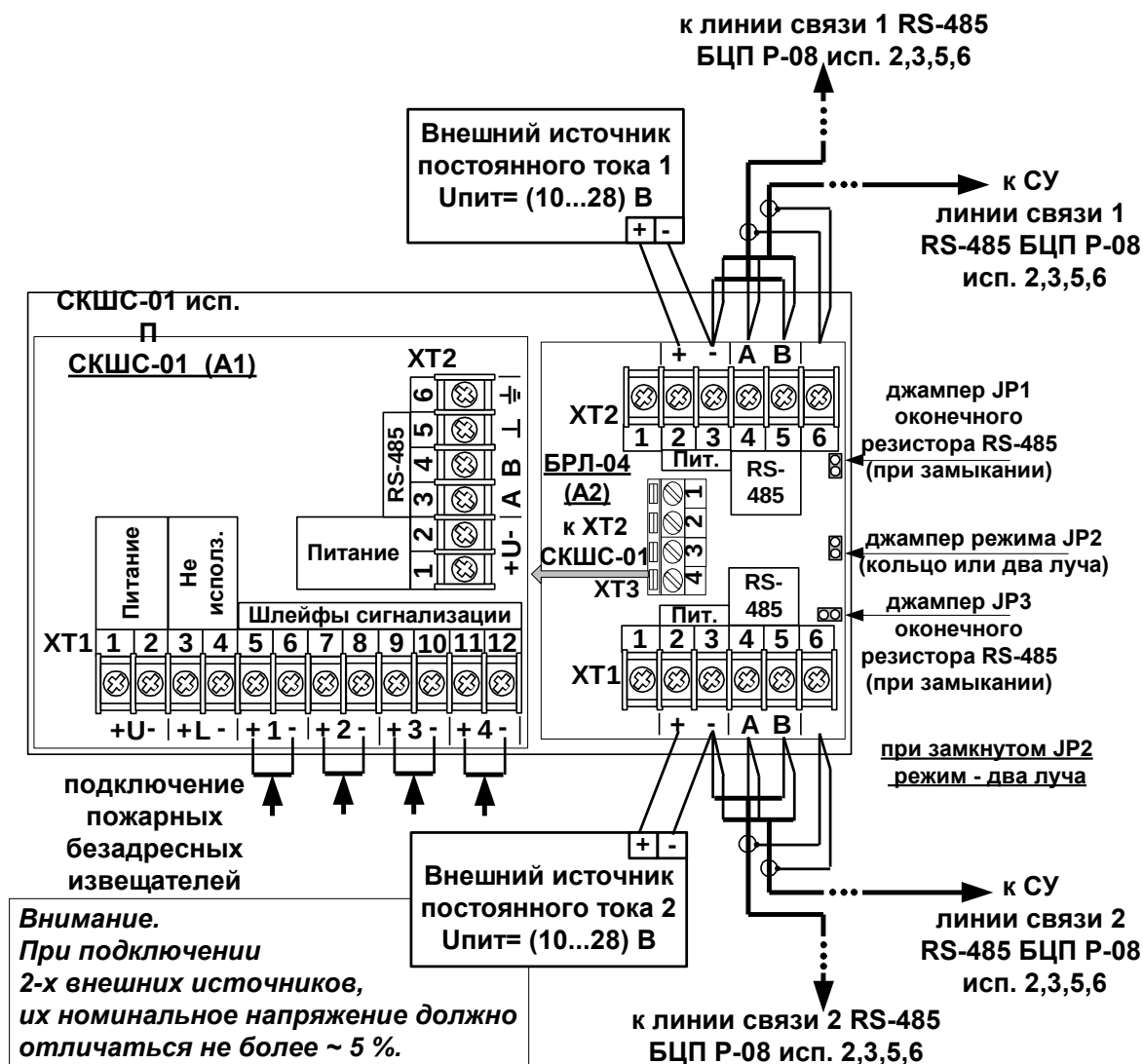
Рис. 1 Применение (подключение) СКШС-01 П в режиме двух параллельных линий связи RS-485 (два луча)
