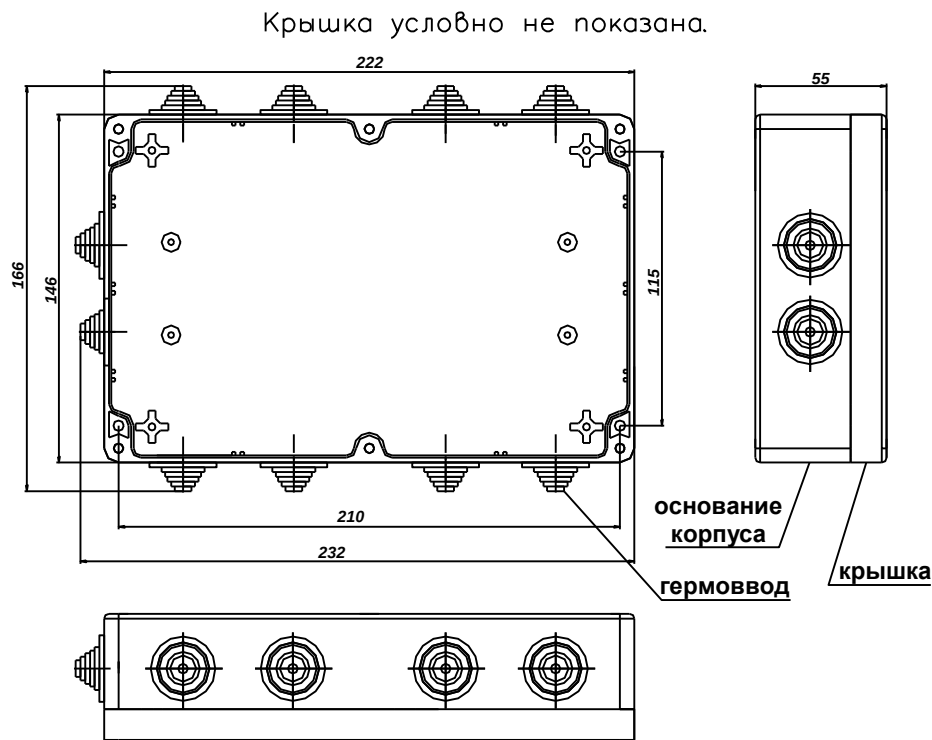
Рис. 16 Габаритные и присоединительные размеры
