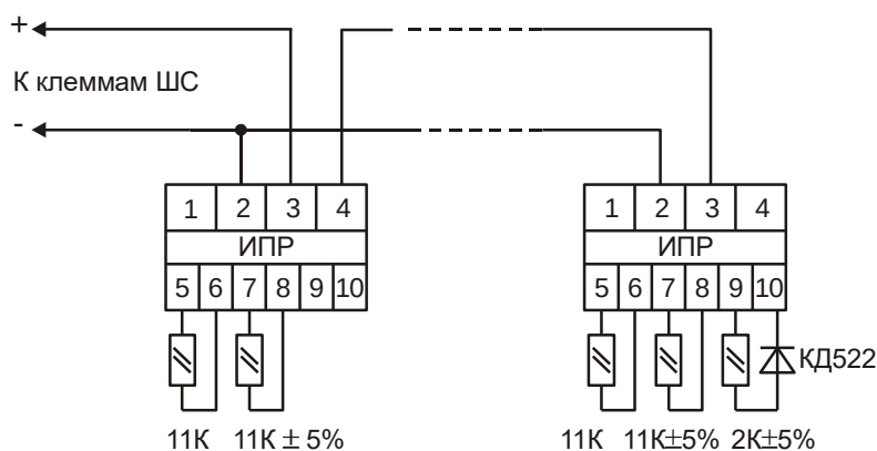
Рис. 12 Схема включения ручного ИП (ИПР и т.п.).
