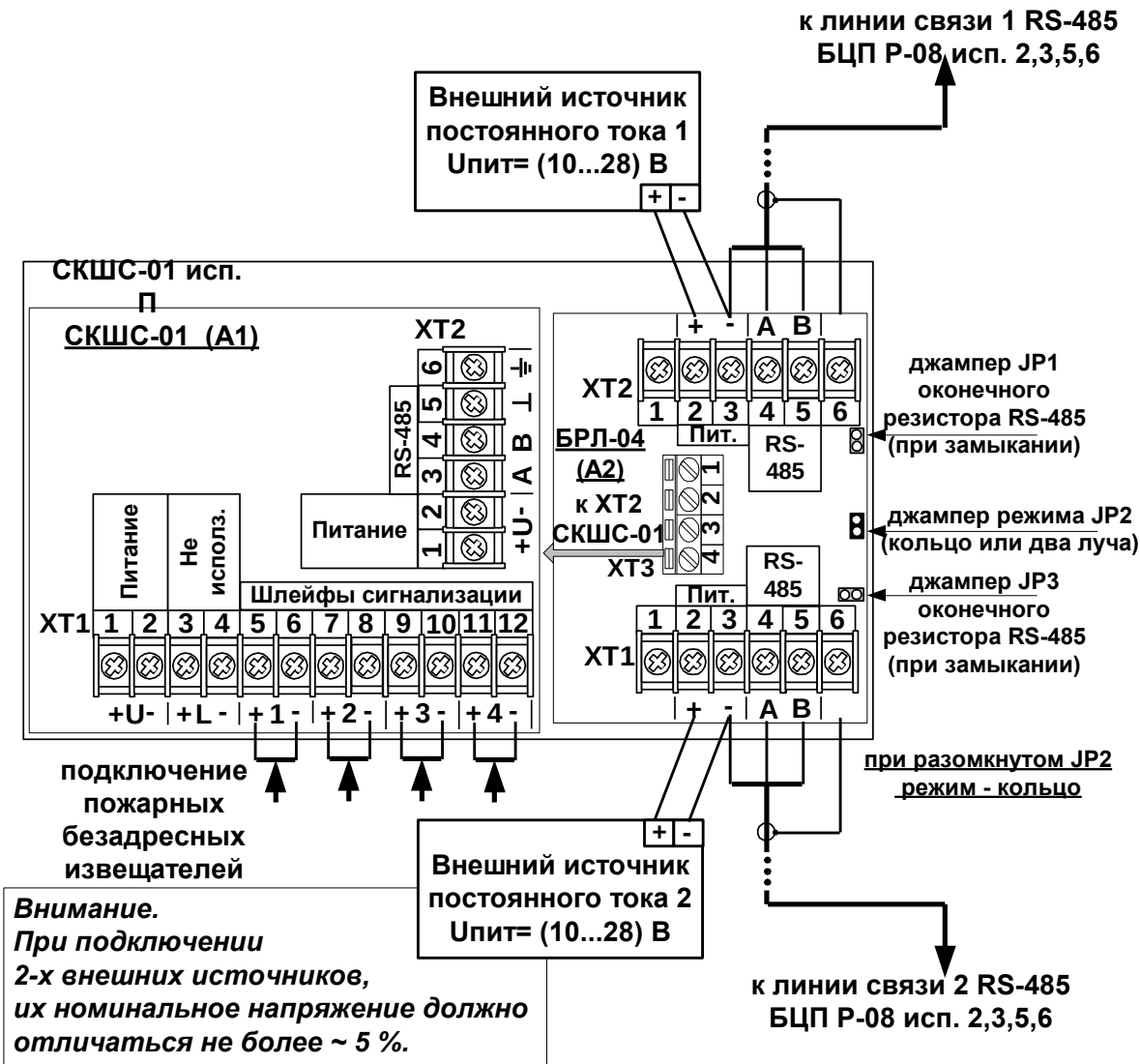
Рис. 2 Применение (подключение) СКШС-01 П в режиме кольца линий связи RS-485
