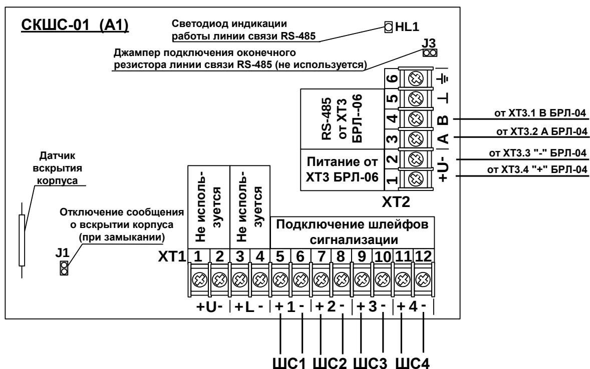
Рис. 17 Подключение модуля СКШС-01(А1)
