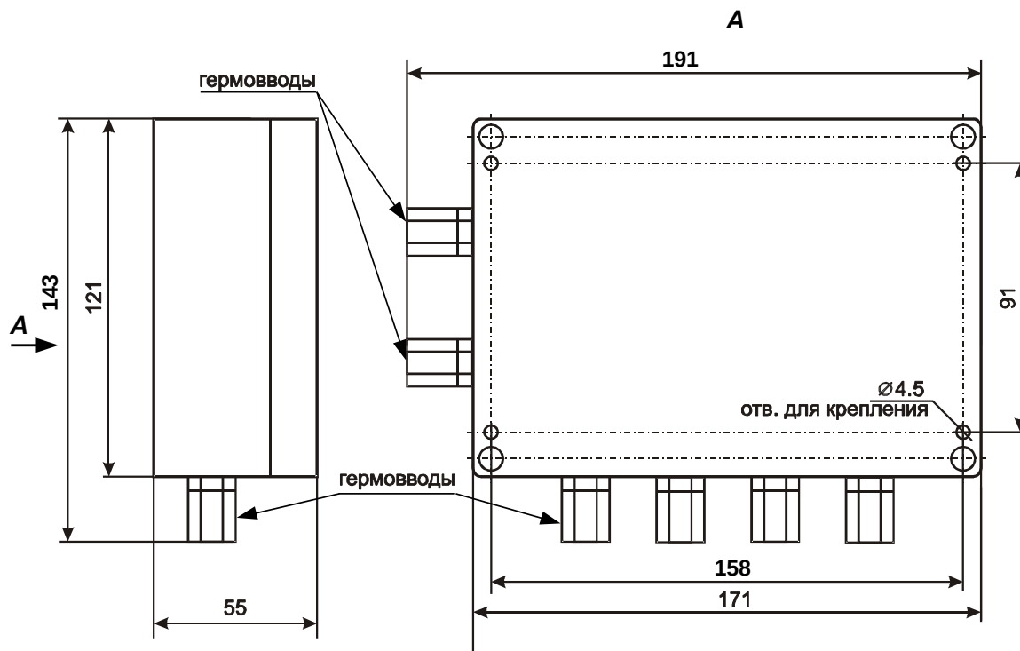
Рис. 16 Габаритные и присоединительные размеры СКШС (исполнение IP65 и индекс K)
