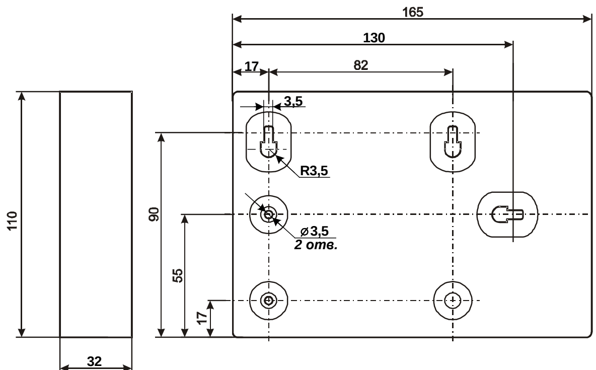
Рис. 4 Габаритные и присоединительные размеры (исполнение IP20)
