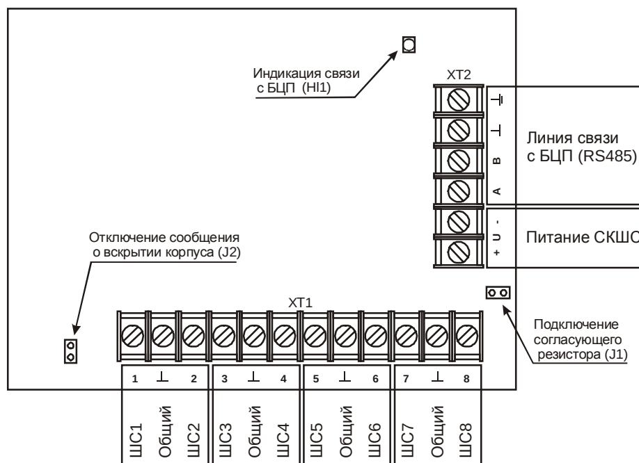
Рис. 6 Подключение СКШС
