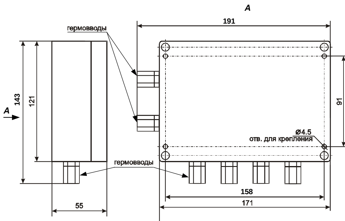
Рис. 5 Габаритные и присоединительные размеры (исполнение IP65 и индекс К)
