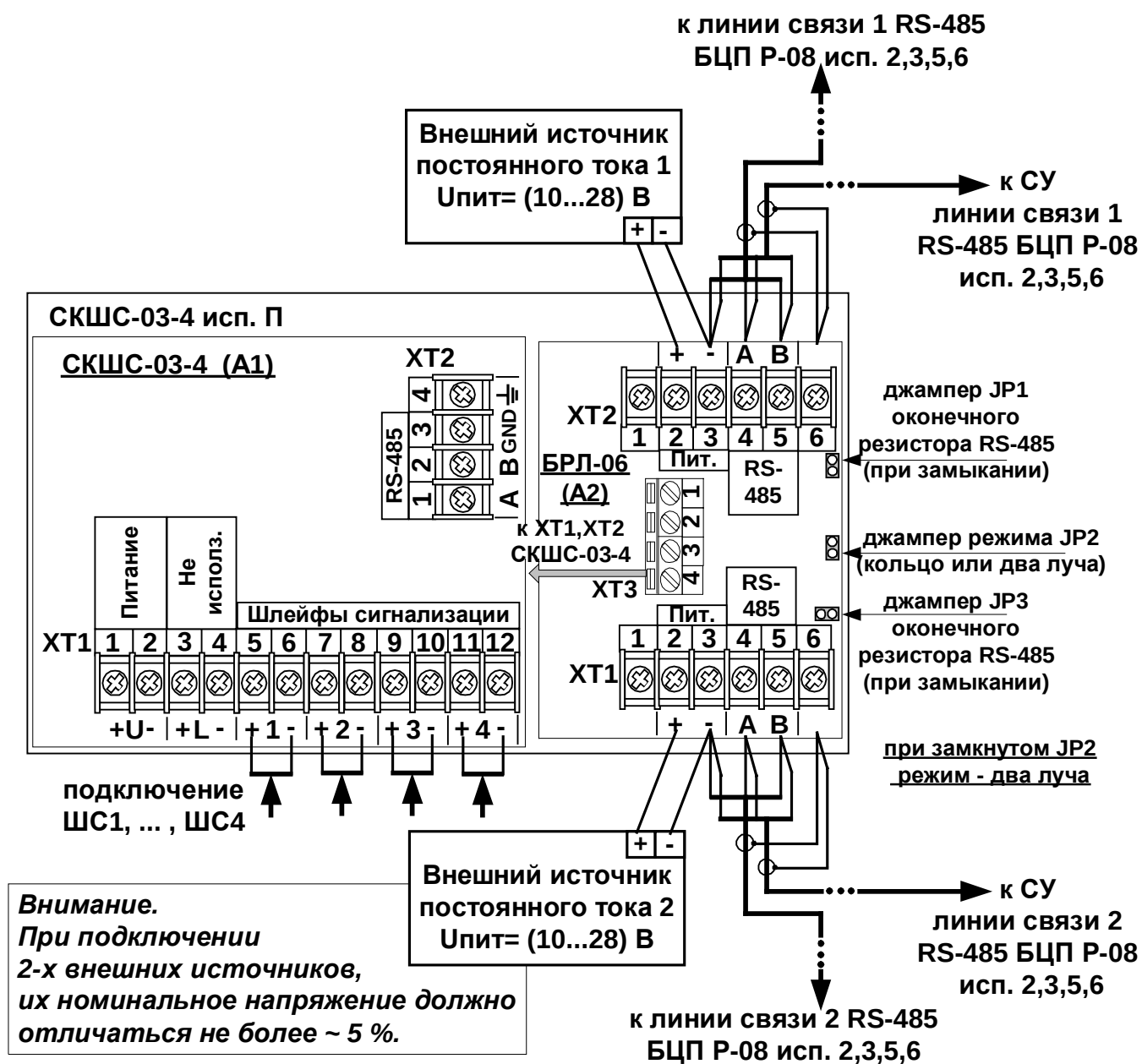
Рис. 1 Применение (подключение) СКШС-03-4 П в режиме двух параллельных линиях связи RS-485 (два луча)
