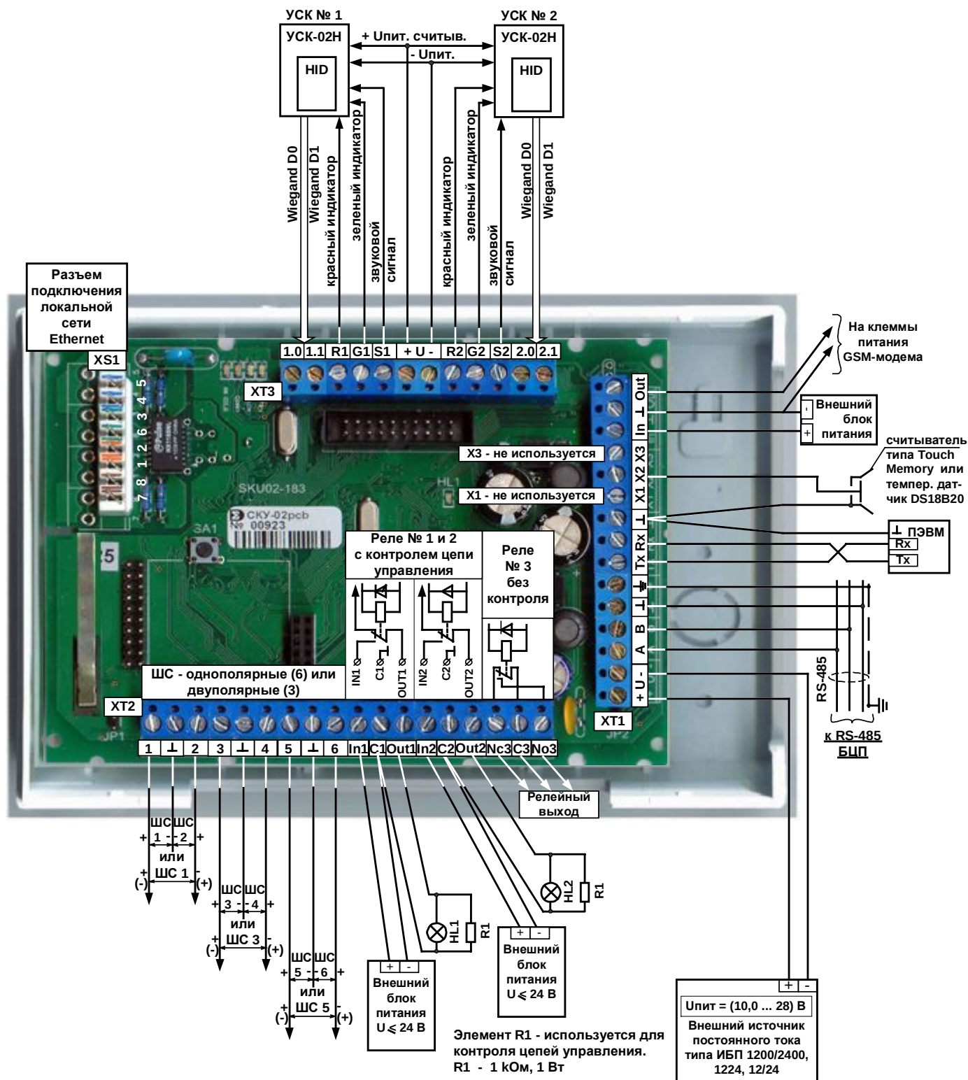
Рис. 3 Подключение СКУ
