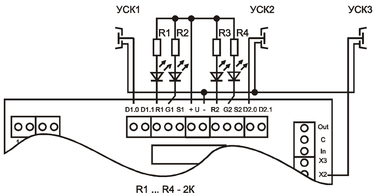
Рис. 20 Подключение светодиодов в качестве индикаторов УСК
