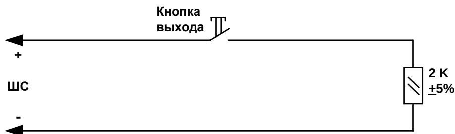
Рис. 17 ШС для приема сообщений о нажатии кнопки выхода
