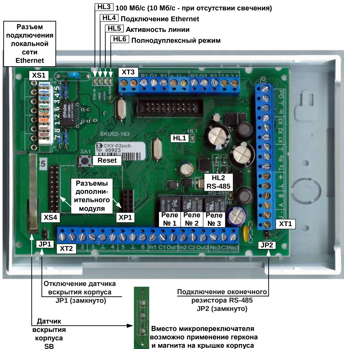
Рис. 1 Внешний вид платы СКУ, расположение элементов
