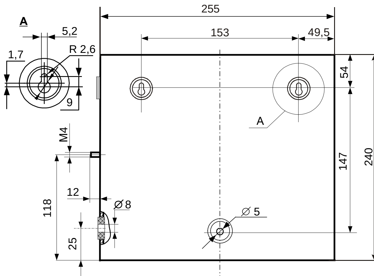
Рис. 27 Габаритные и присоединительные размеры СКУ-02 (исп. 1)
