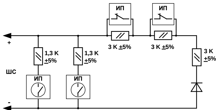
Рис. 15 Подключение извещателей к двухполярному ШС
