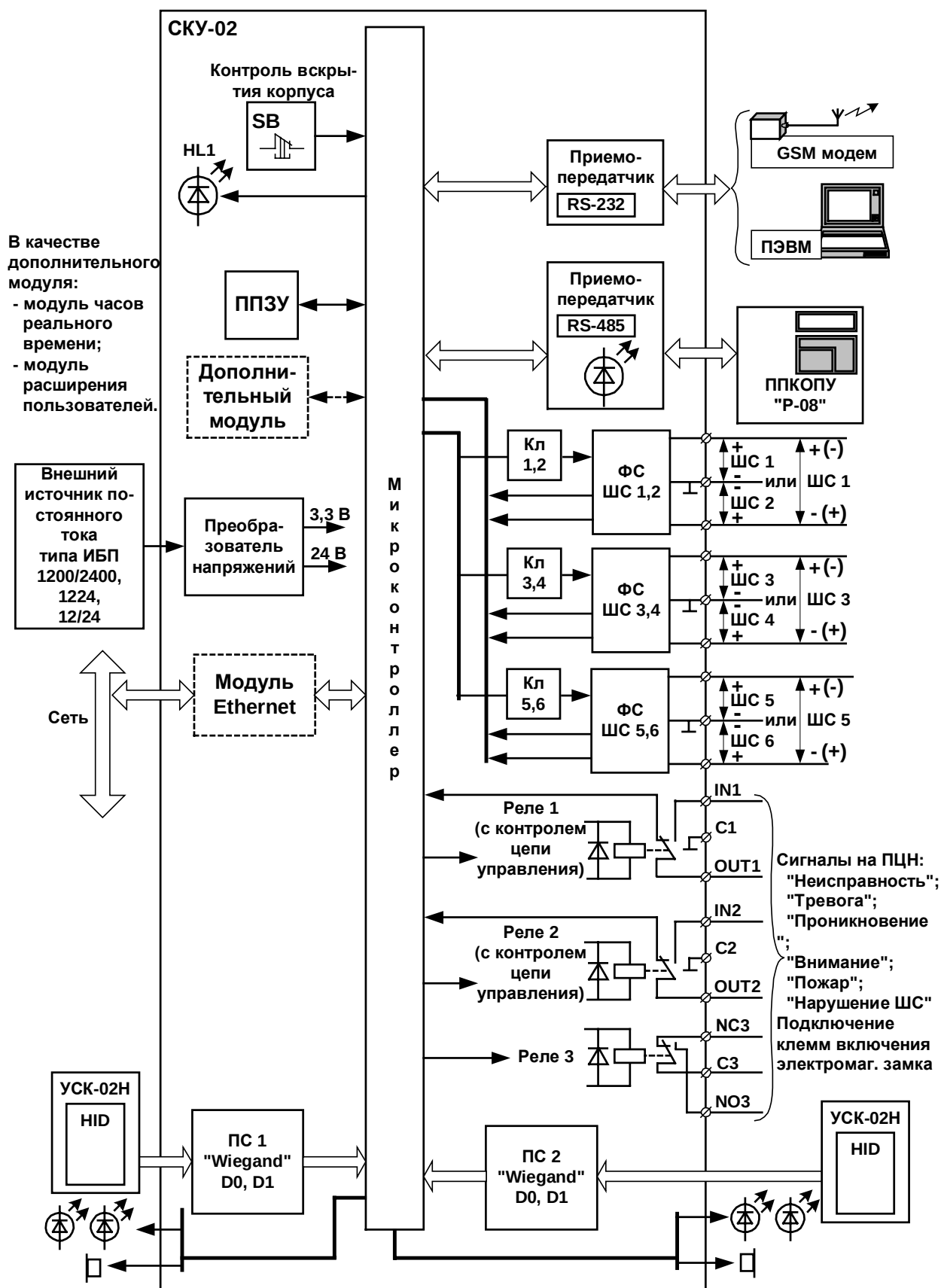
Рис. 2 Схема структурная СКУ
