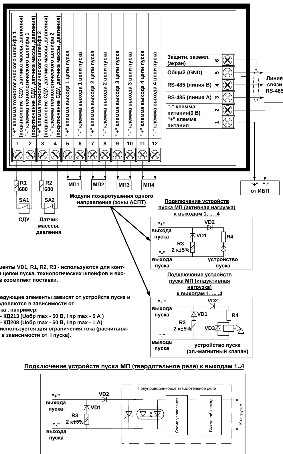
Рис. 6 Схема подключения СКУП-01 (A1)
