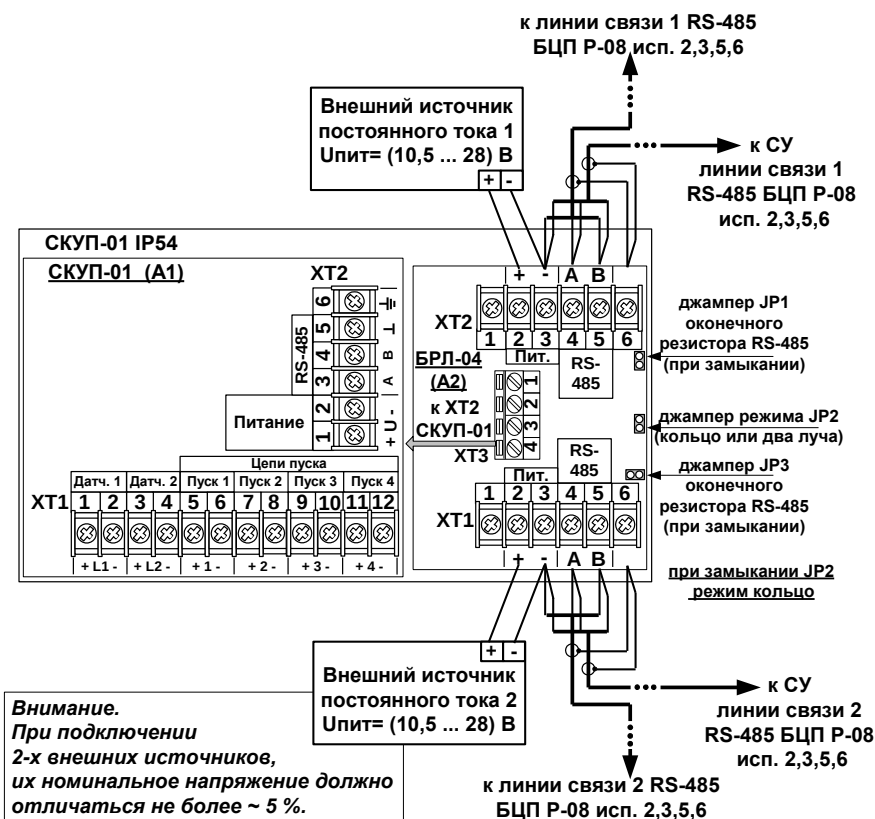
Рис. 2 Применение (подключение) СКУП-01 IP54 в режиме двух радиальных линиях связи RS-485 (два луча)
