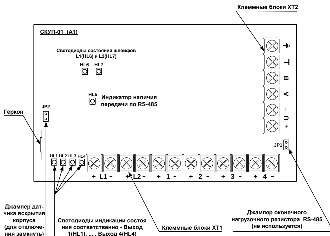
Рис. 4 Внешний вид с обозначением элементов модуля СКУП-01 (А1)
