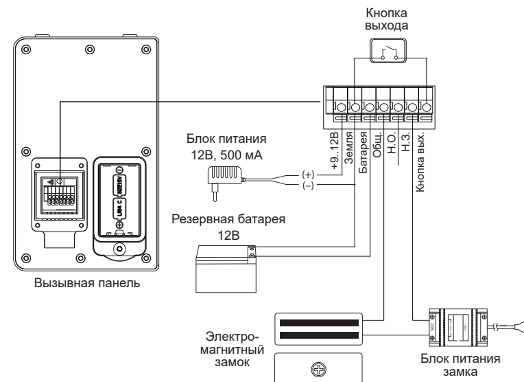
Схема 2. Подключение электромагнитного замка к вызывной панели.
