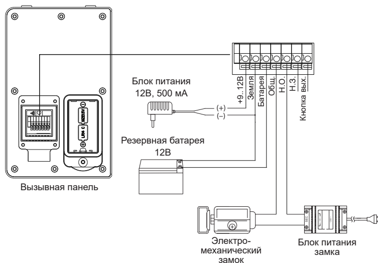
Схема 1. Подключение электромеханического замка к вызывной панели.
