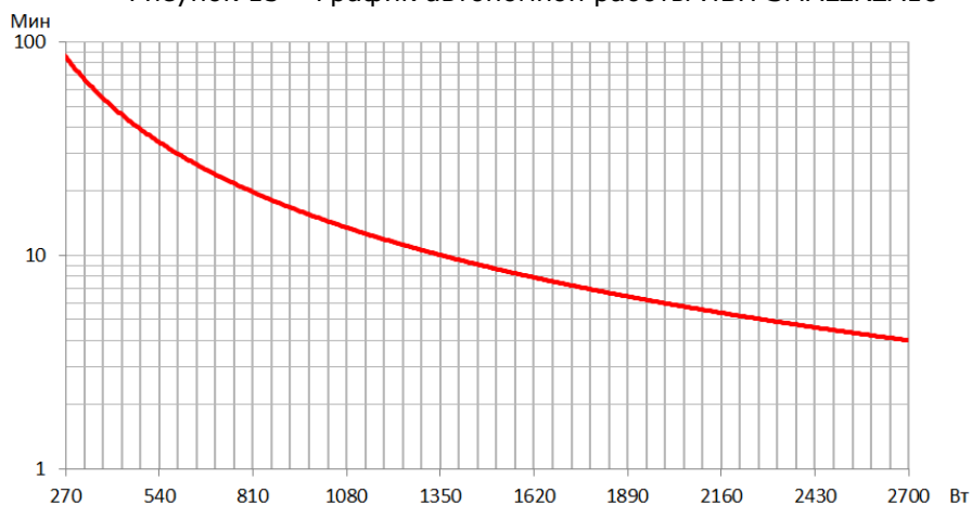
Рисунок 16 – График автономной работы ИБП SMALLR3A5
