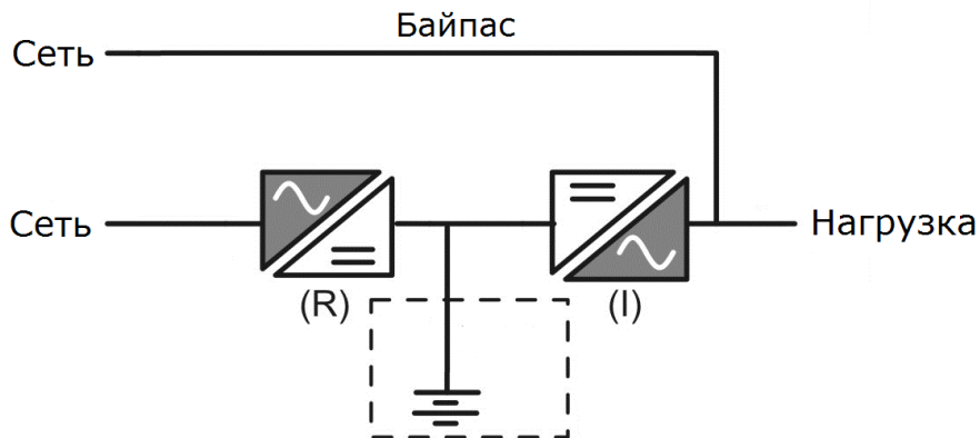
Рисунок 2 - Блок-схема
