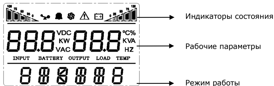
Рисунок 9 – Экран ИБП
