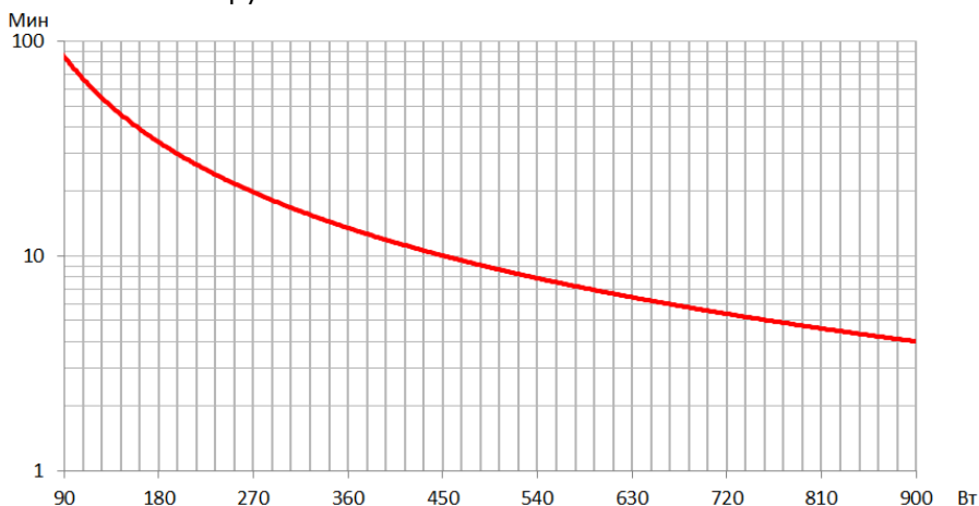
Рисунок 12 – График автономной работы ИБП SMALLR1A5
