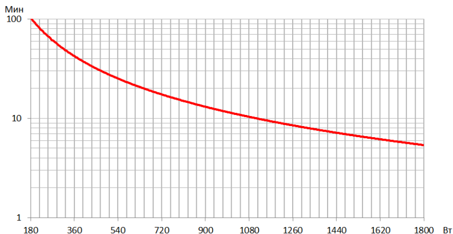
Рисунок 15 – График автономной работы ИБП SMALLR2A10
