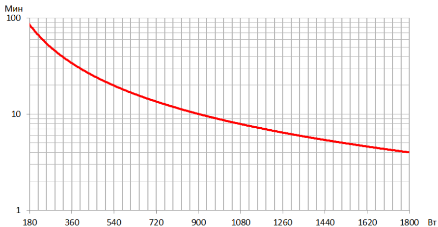
Рисунок 14 – График автономной работы ИБП SMALLR2A5
