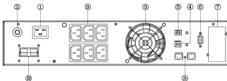
Figura 3 - Pannello posteriore dell'UPS SMALLT1 e SMALLT2 / SMALLT3
