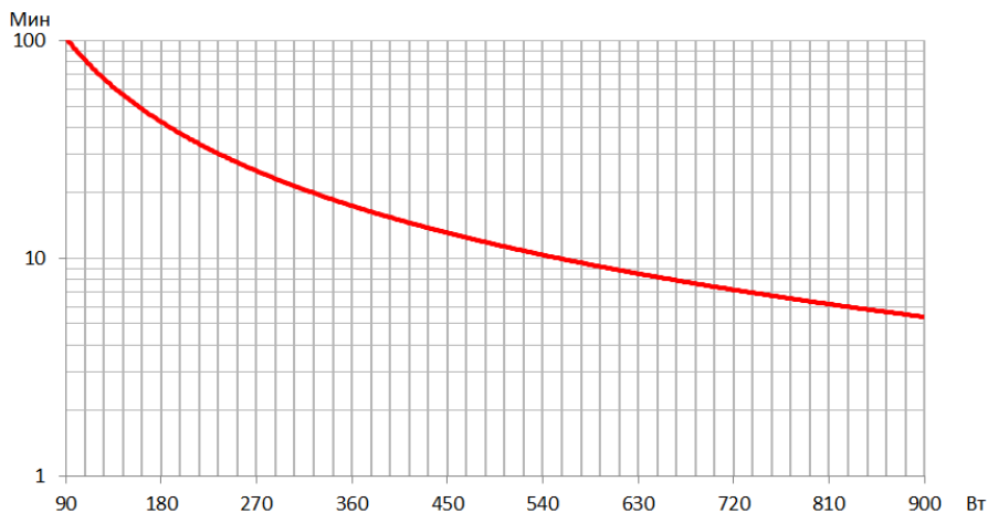
Рисунок 13 – График автономной работы ИБП SMALLR1A10
