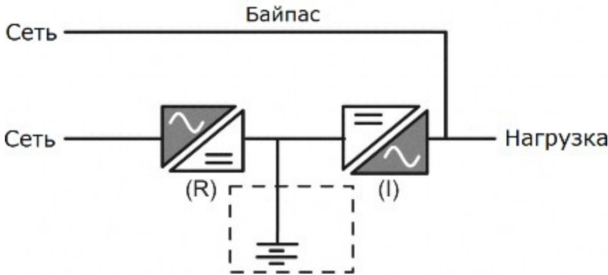
Рис. 2. Блок-схема
