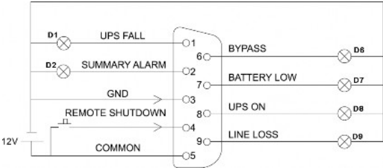
Рис. 7. Отображение состояния ИБП с помощью разъема DB-9
