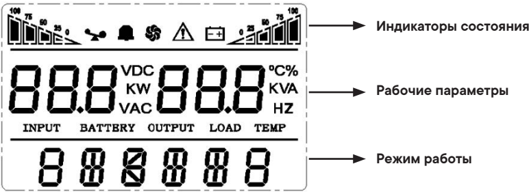
Рис. 9. Отображение параметров на экране ИБП
