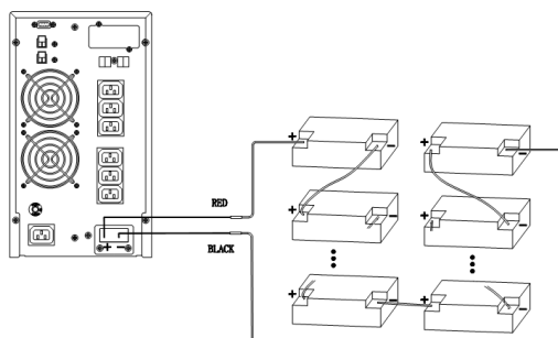
Рис. 4. Схема подключения внешних батарей.
