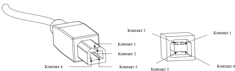
Тип соединения «штекер» Тип соединения «гнездо»
