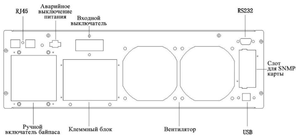
ИБП SMARTWATT UPS SECURE 6kVA L, вид сзади.
