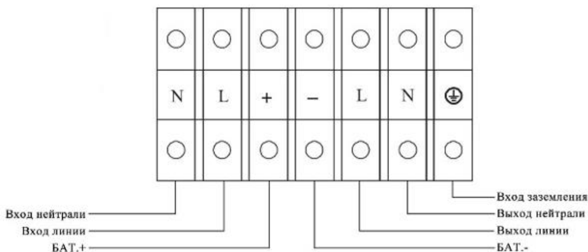
Схема подключения клеммного блока входа и выхода для моделей UPS SECURE 6-10kVA L
