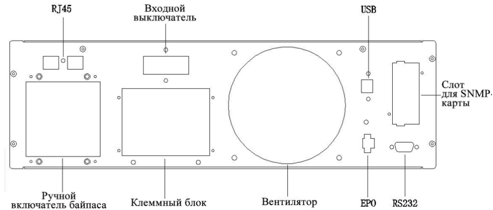
ИБП SMARTWATT UPS SECURE 6kVA L, вид сзади.
