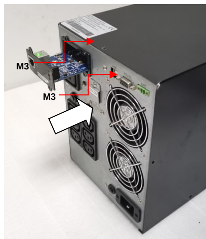
Карта Megatec SNMP – CY504B
