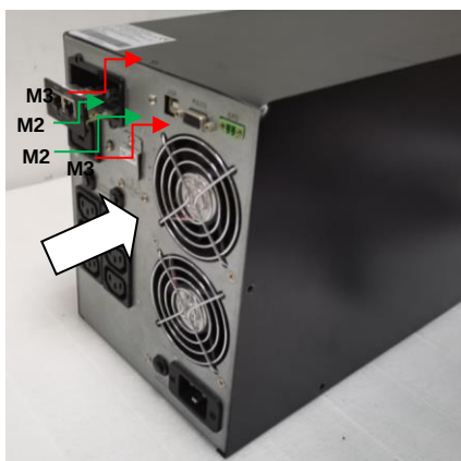
SNMP MINI CARD 3
