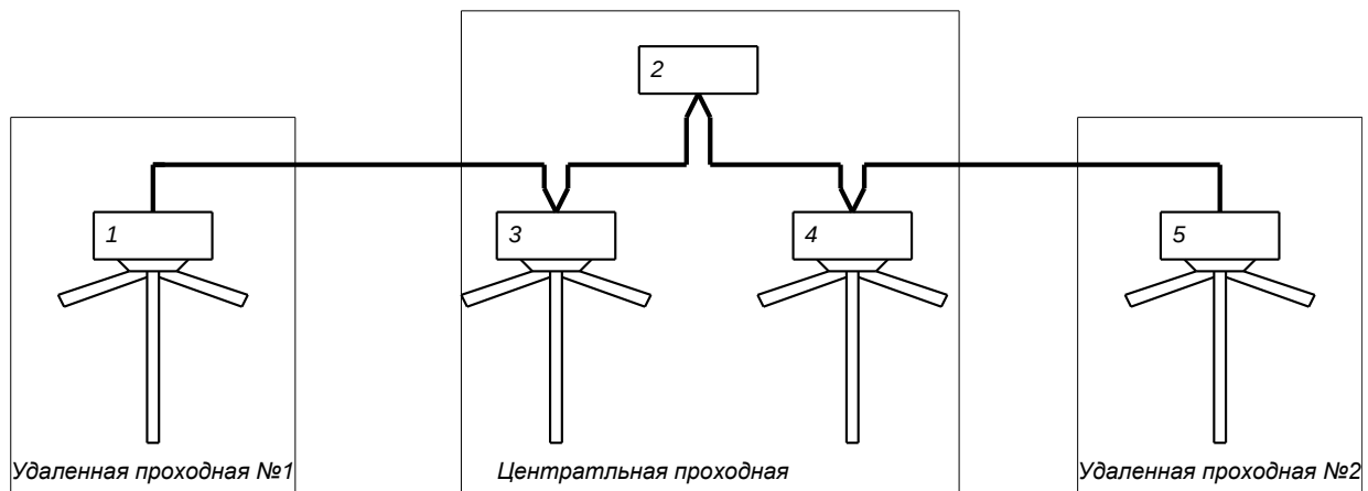
Рисунок 2.4.2 – Пример размещения оборудования
