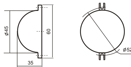
Рис.1. Габаритные и установочные размеры оповещателя
