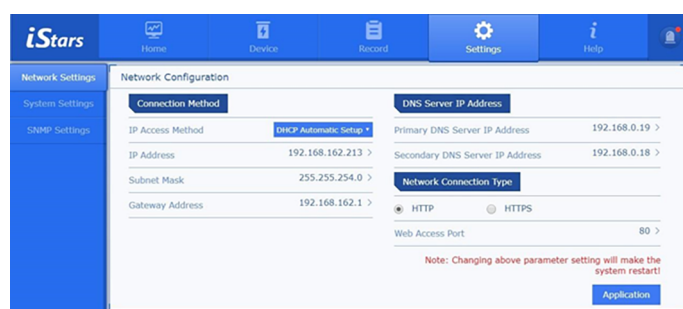
Рис. 3.17. Конфигурация сети
