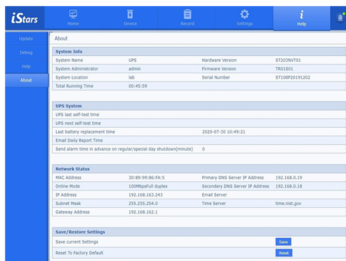
Рис. 3.26. О программе
