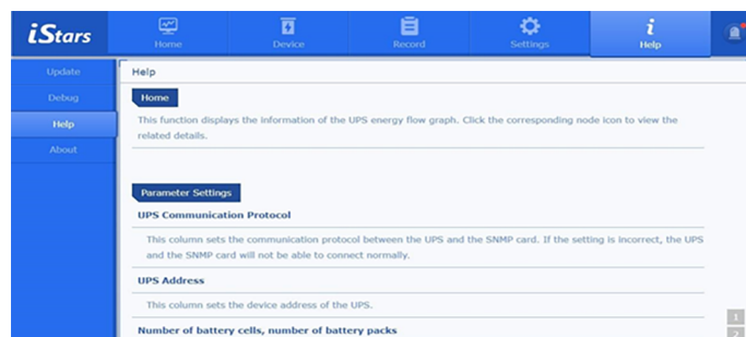
Рис. 3.25. Страница помощи
