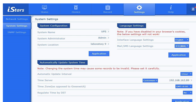
Рис. 3.19. Системные настройки
