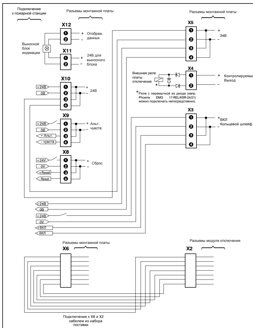
Рис. 5.21: Подключение модуля отключения
