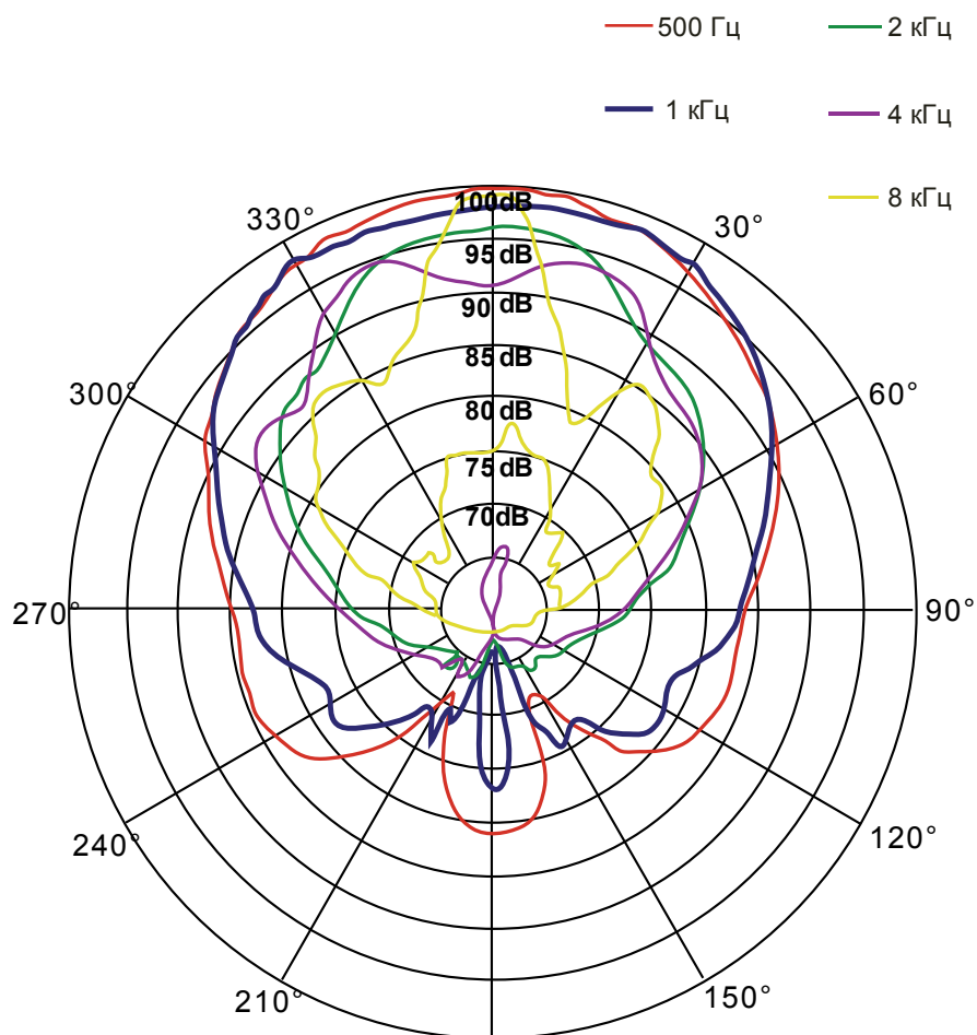
Рисунок 2 – Диаграмма направленности громкоговорителя.
