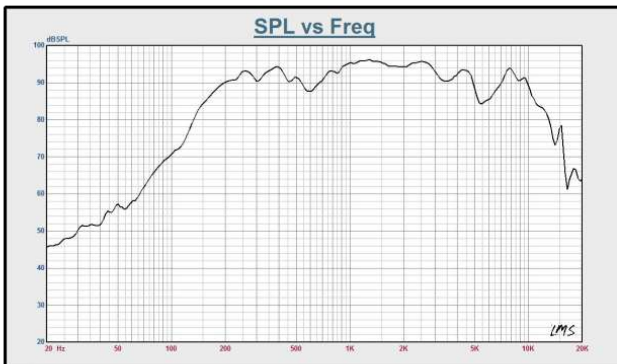
Рисунок 3 - Амплитудно-частотная характеристика SCS-830
