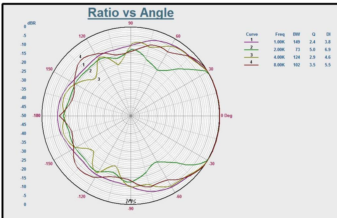
Рисунок 4 – Диаграмма направленности громкоговорителя SHS-20TA
