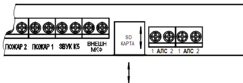
Рисунок 3.10 - Направление подачи SD-карты в держатель
