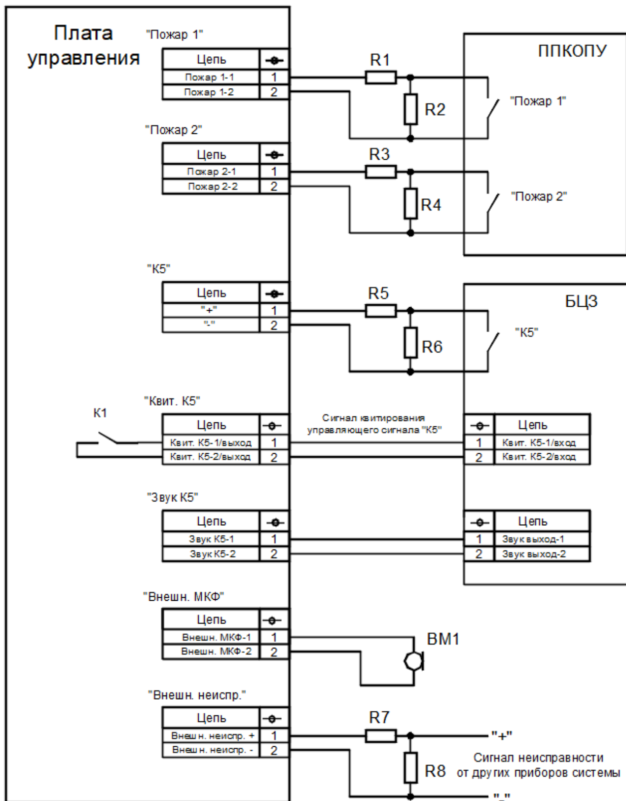
б) Соединение ППУ с ППКОПУ и БЦЗ
