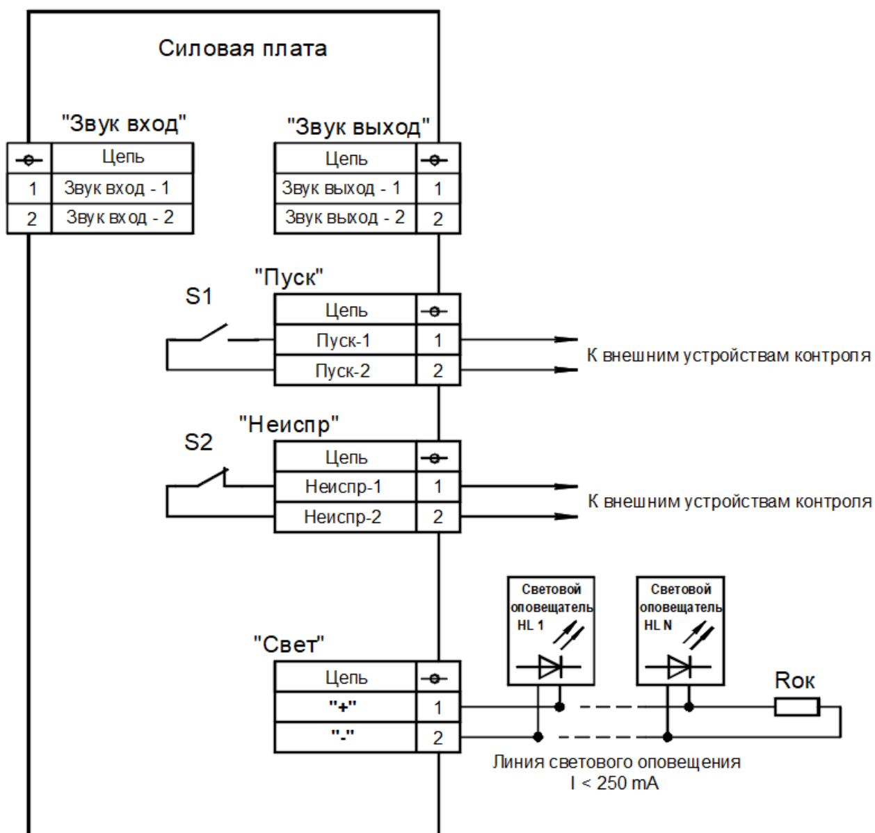
Рисунок 3.2 - Схема соединения силовой платы ППУ с внешними устройствами
