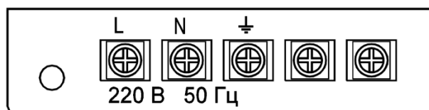
Рисунок 3.3 - Расположение колодок зажимов сетевого блока питания ППУ
