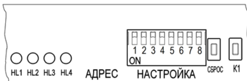
Рисунок 3.8 - Общий вид блока переключателей НАСТРОЙКА
