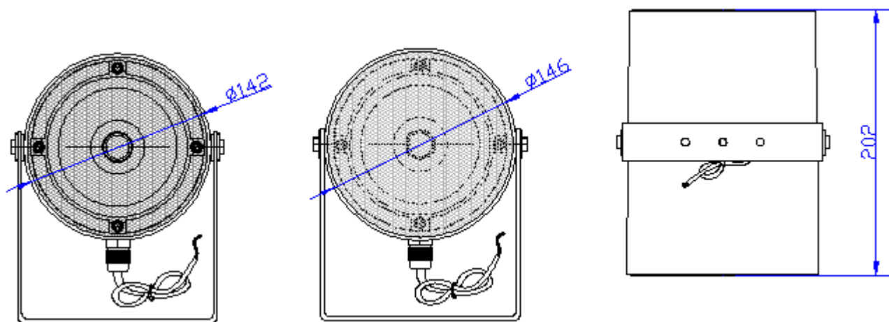
Рисунок 7 – Габаритные и установочные размеры SNS-20
