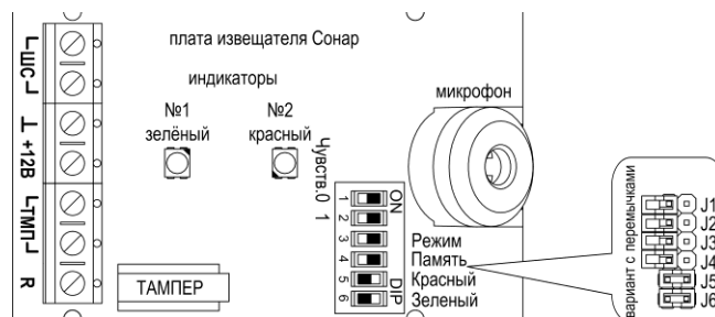
Рис.1 Плата извещателя
