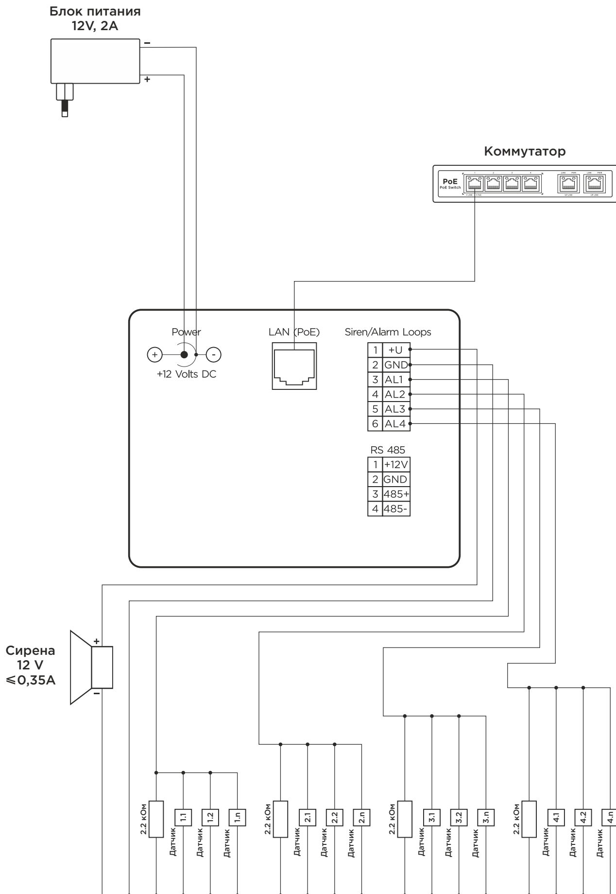
Схема подключения датчиков охранной сигнализации
