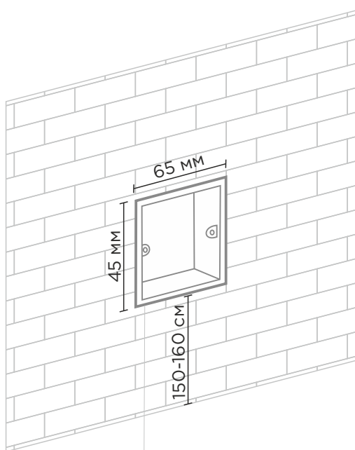
Монтажная коробка
