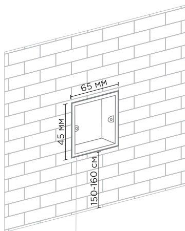
Монтажная коробка
