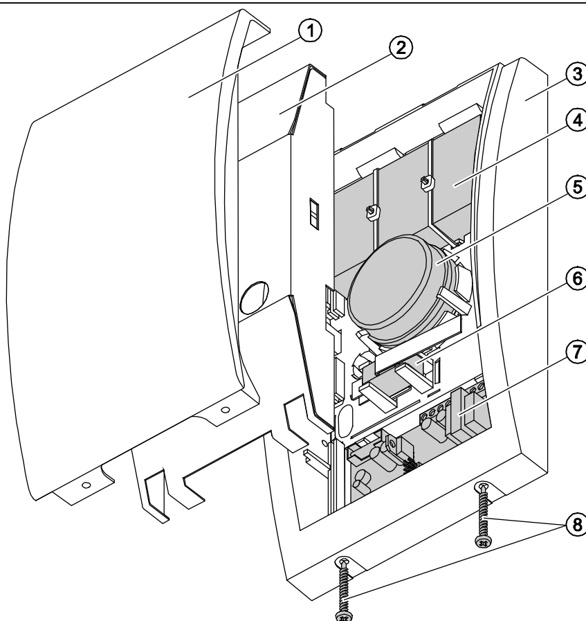
Рис. 1. Вид оповещателя.
