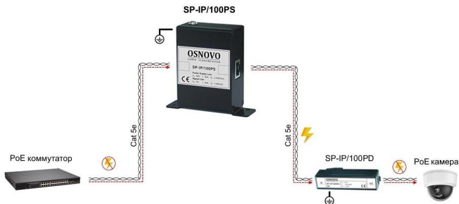
Рис.6 Схема подключения устройства грозозащиты на примере SP-IP/100PS, SP-IP/100PD.
