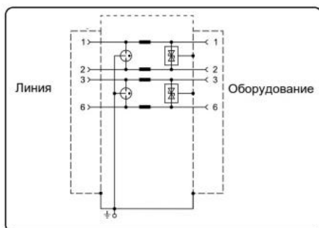
Рис.4 Внешний вид и электрическая схема SP-IP4/100
