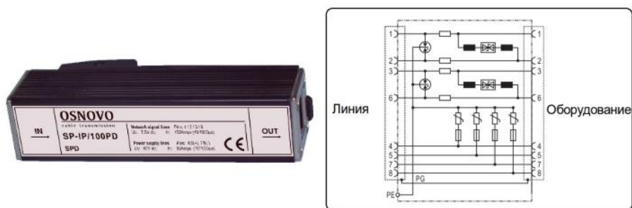
Рис.2 Внешний вид и электрическая схема SP-IP/100PD.
