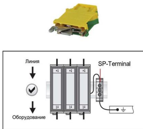
Рис.8 SP-Terminal. Внешний вид. Монтаж.
