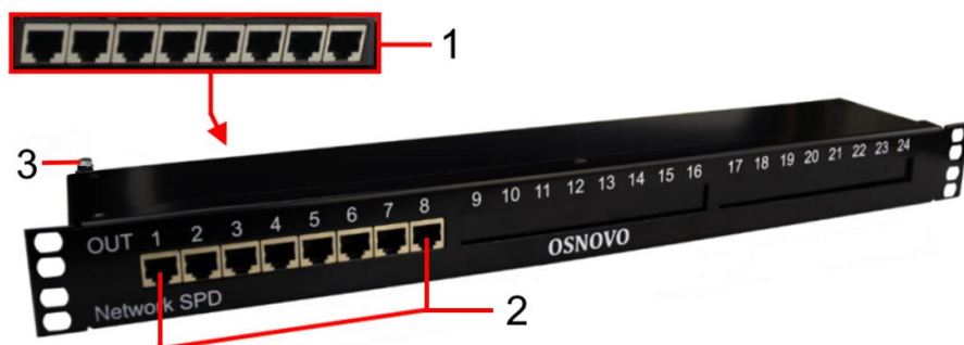
Рис.3 Разъёмы устройств грозозащиты на примере SP-IP8/100R.
