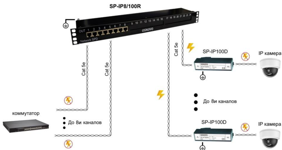
Рис.4 Схема подключения устройства грозозащиты на примере SP-IP8/100R.
