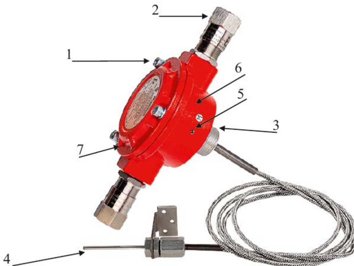
1 – винт М6 с шайбой; 2 – кабельный ввод; 3 – резьба под гайку М30х1,5; 4 – чувствительный элемент; 5 – светодиодный индикатор; 6 – корпус извещателя; 7 – крышка извещателя. Рисунок 3 – Извещатель Спектрон-101-Exd-ВЭ
