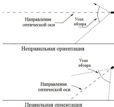
Рисунок 4 – Установка извещателя по отношению к горизонту
