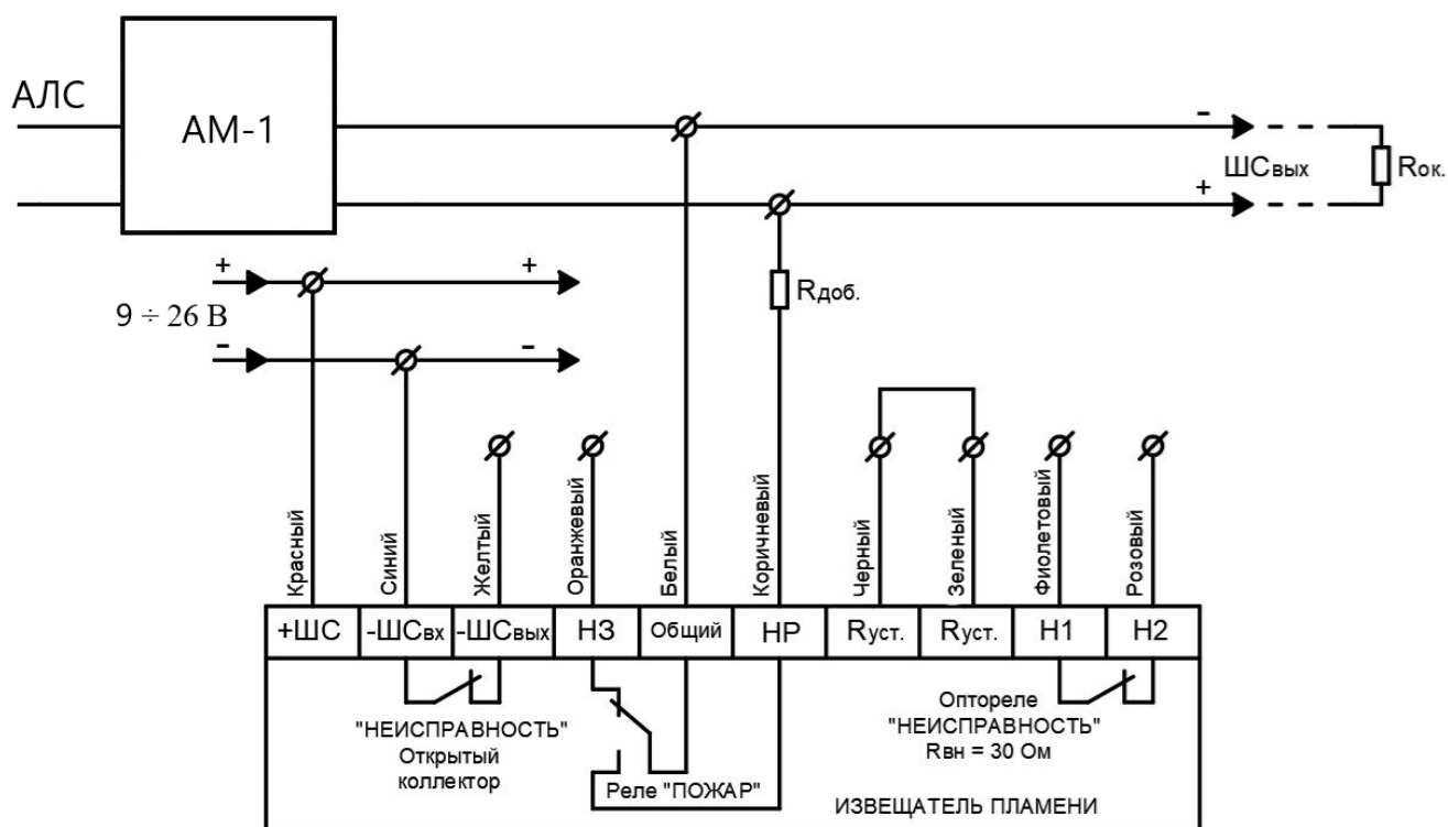
Рисунок Б8 – 4-х проводная схема подключения Спектрон-205 к АМ-1 без использования режима «НЕИСПРАВНОСТЬ»
