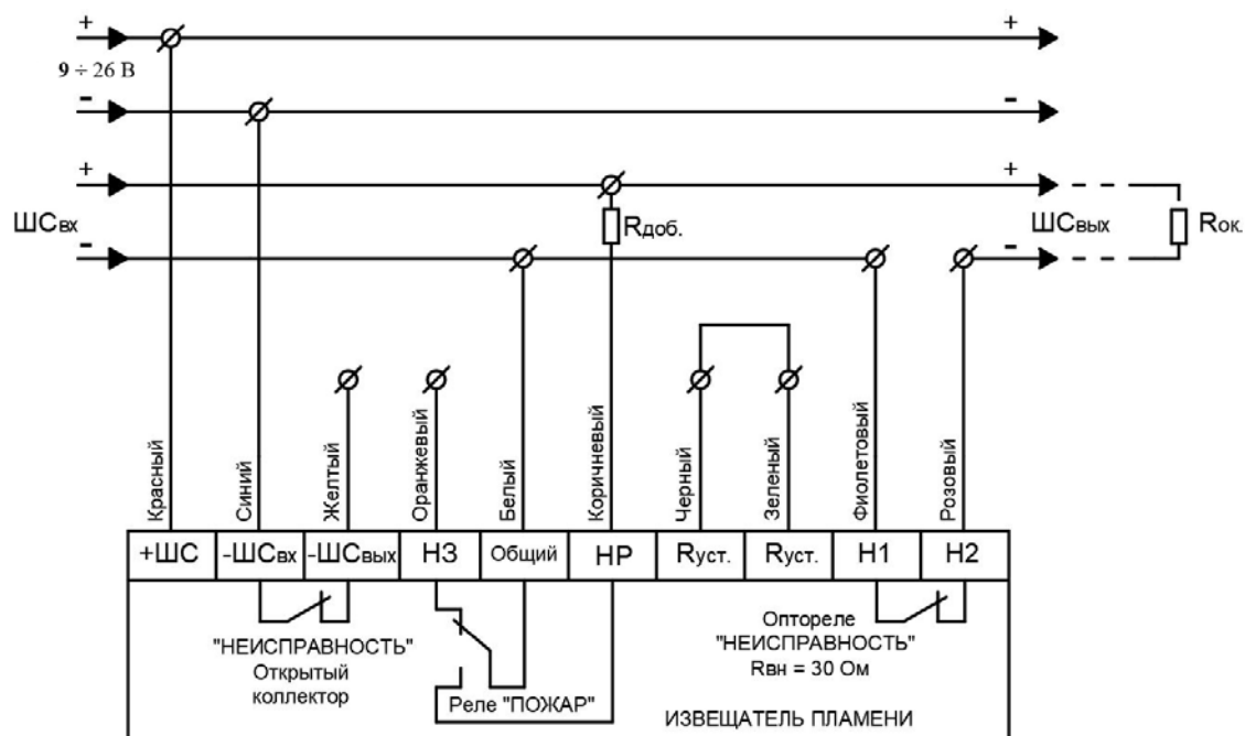
Рисунок Б3 – 4-х проводная схема подключения Спектрон-205 с использованием режима «НЕИСПРАВНОСТЬ»
