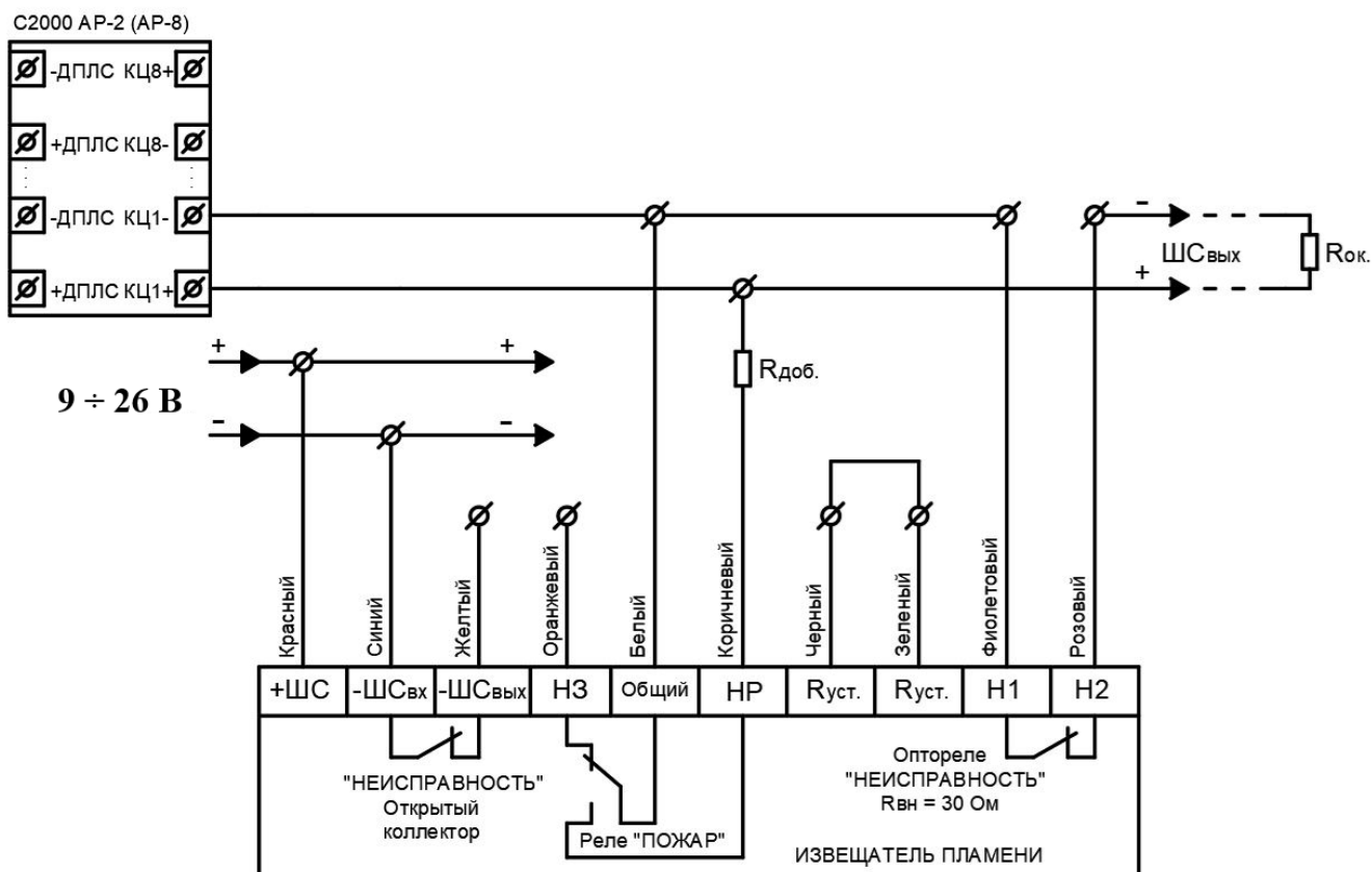
Рисунок Б5 – 4-х проводная схема подключения Спектрон-205 к С2000-АР2 (АР-8) с использованием режима «НЕИСПРАВНОСТЬ»
