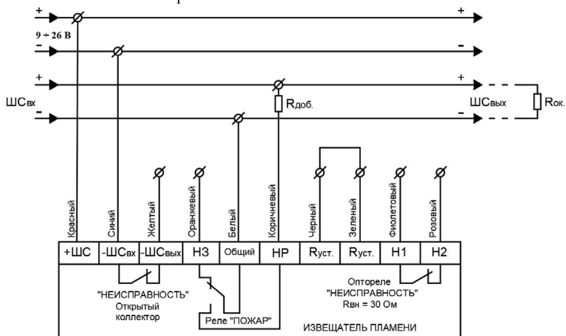
Рисунок Б4 – 4-х проводная схема подключения Спектрон-205 без использования режима «НЕИСПРАВНОСТЬ»
