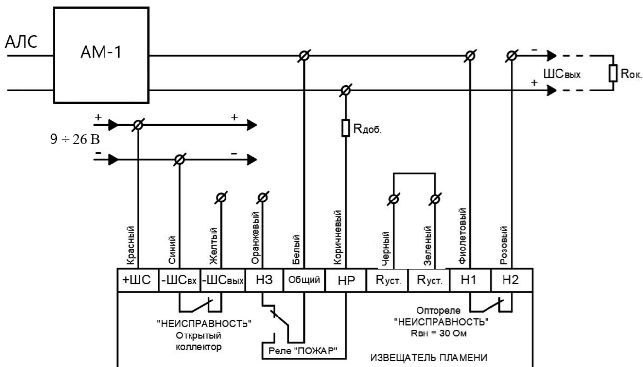
Рисунок Б7 – 4-х проводная схема подключения Спектрон-205 к АМ-1 с использованием режима «НЕИСПРАВНОСТЬ»
