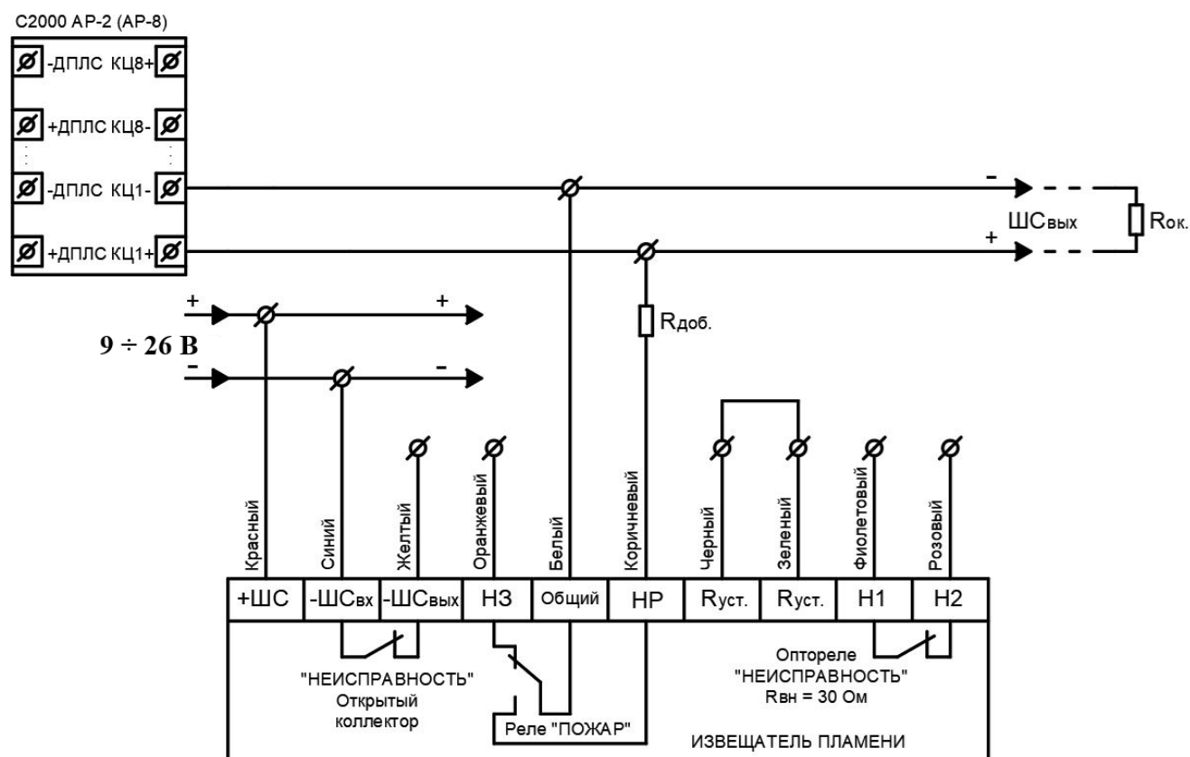
Рисунок Б6 – 4-х проводная схема подключения Спектрон-205 к С2000-АР2 (АР-8) без использования режима «НЕИСПРАВНОСТЬ»
