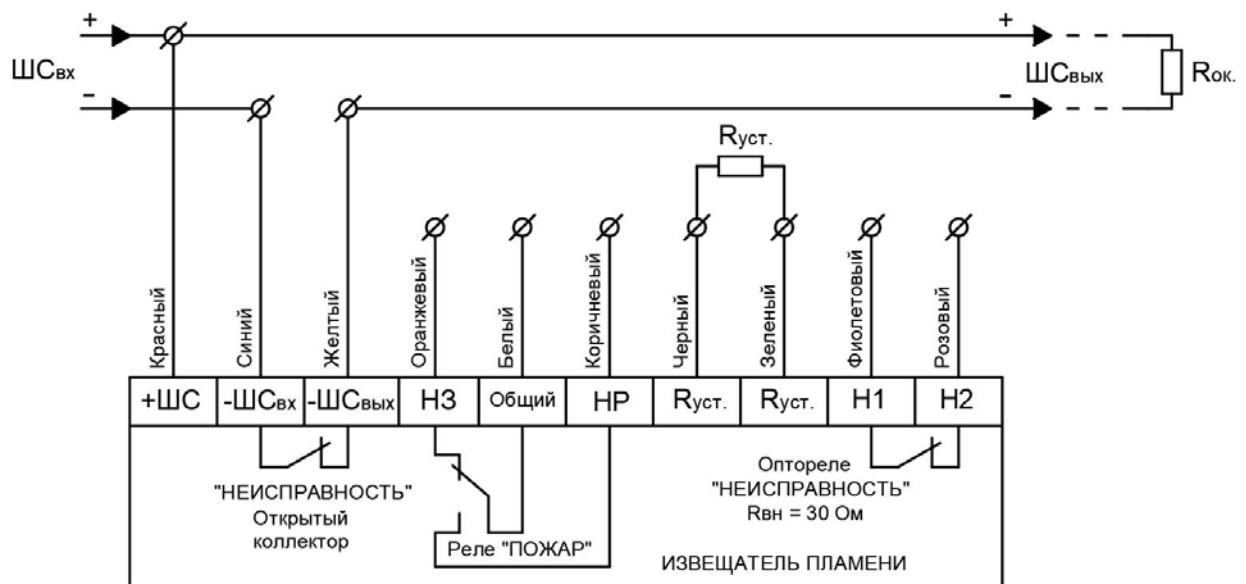
Рисунок Б1 – 2-х проводная схема подключения Спектрон-205 с использованием режима «НЕИСПРАВНОСТЬ»
