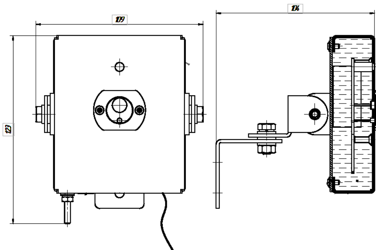
Рисунок А2 – Габаритные и установочные размеры Спектрон-205-М-Н
