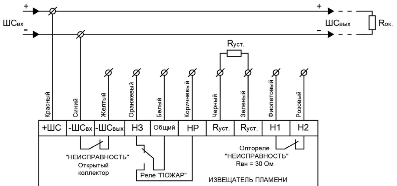
Рисунок Б2 – 2-х проводная схема подключения Спектрон-205 без использования режима «НЕИСПРАВНОСТЬ»
