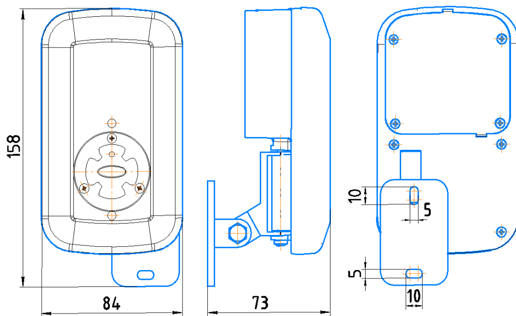
Рисунок А1 – Габаритные размеры Спектрон-401-Ехi, -401.01-Ехi, -401-Exm, -401.01-Exm
