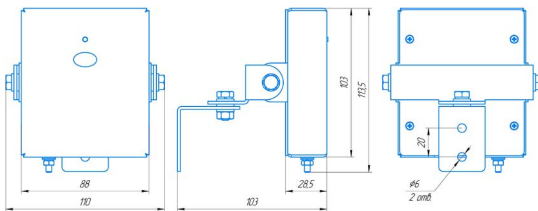
Рисунок А2 – Габаритные размеры Спектрон-401-М, -401-Ехi-М, -401.01-Ехi-М, -401-Exm-М, -401.01-Exm-М
