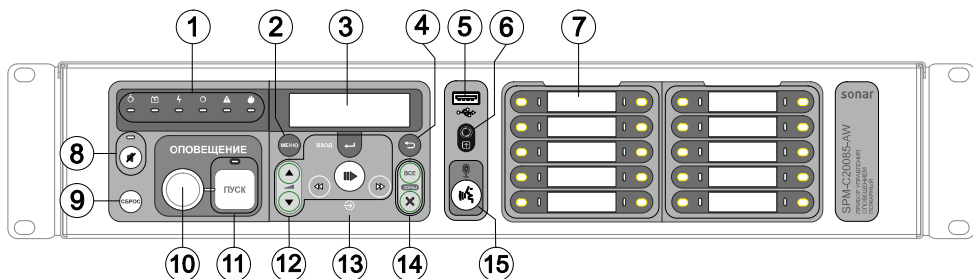
Рисунок 5 – Лицевая панель моделей Sonar SPM-C20xxx-xx (20 зон)
