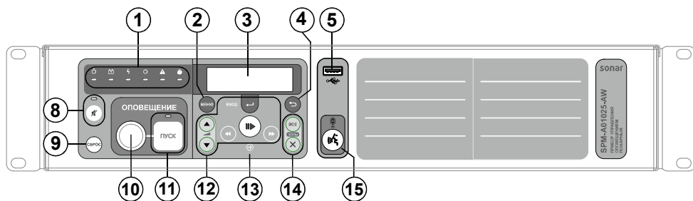
Рисунок 2 – Лицевая панель моделей Sonar SPM-A01xxx-xW (1 зона)
