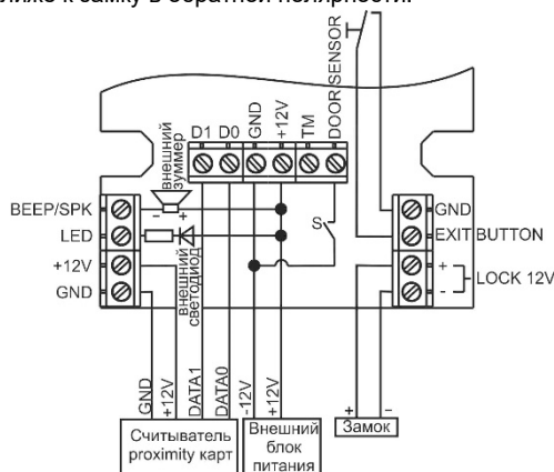
Рисунок 2 - Схема подключения.
