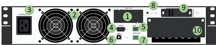
Рисунок 7-2. Задняя панель (Модуль ИБП)
