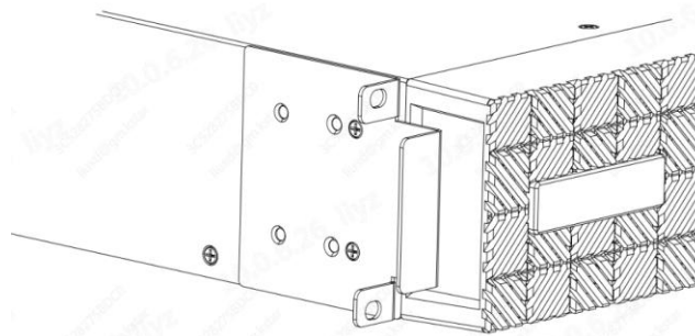
Рисунок 9-2. Монтажные отверстия
