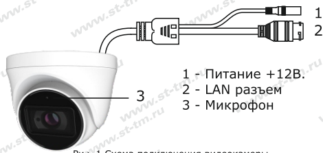
Рис. 1 Схема подключения видеокмеры
