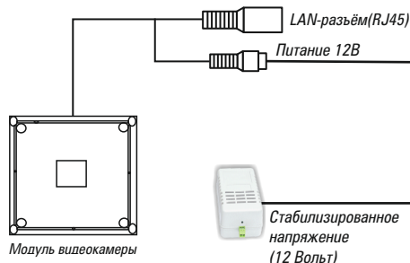
Рис.1 Схема подключения
