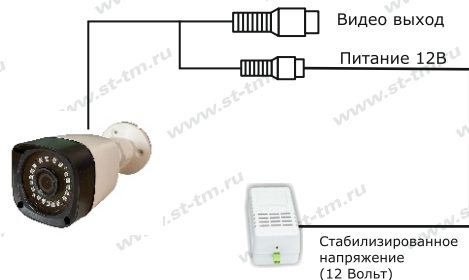
Рис.1 Схема подключения
