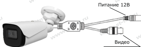
Рис.1 Схема подключения
