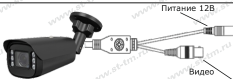
Рис.1 Схема подключения
