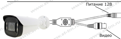
Рис.1 Схема подключения
