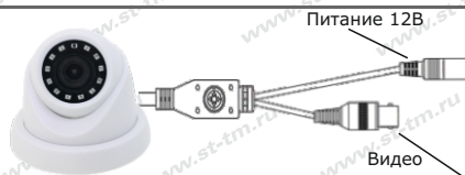
Рис.1 Схема подключения
