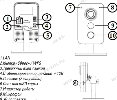
Рис. 1 Схема подключения
