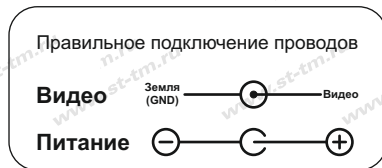
Рис.2 Подключение разъемов
