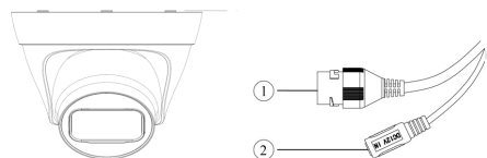
1- LAN + PoE; 2 - Питание 12В.
