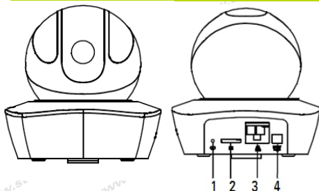
1 - Кнопка «Сброс», 2 - Слот для карты microSD, 3 - LAN, 4 - Стабилизированное питание 5В
