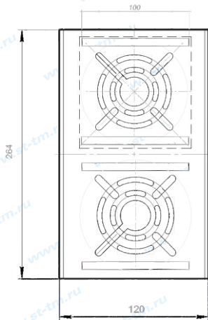
Рис.1 Габаритные размеры
