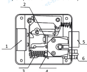
Рис.2. Внутренняя конструкция замка
