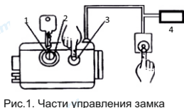
Рис.1. Части управления замка
